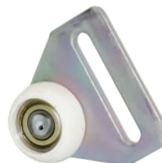
11069 ΡΟΔΑΚΙΑ PB ΓΙΑ ΡΑΓΑ 400 RUNNERS PB FOR RAIL 400 b=29 / d=37 / L=62 / A=52
