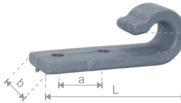
11008 ΠΙ PB TIR ΤΕΤΡΑΓΩΝΟ ΜΙΚΡΟ STAPLES PB TIR SQUARE SMALL a=34 / h=11
