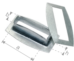
11001 ΚΑΨΟΥΛΕΣ ΡΒ ΟΡΘΟΓΩΝΙΕΣ ΣΙΔΕΡΕΝΙΕΣ EYELETS PB RECTANGULAR IRON a=27 / h=8 / b=10,5
