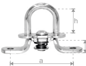
11007 ΠΙ PB ΓΥΡΙΣΤΟ ΜΕ ΕΛΑΤΗΡΙΟ STAPLES PB TIR ROUNDED SPRING a=51 / h=12 / H=27
