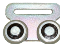
11076 ΡΟΔΑΚΙΑ PB ΔΙΠΛΑ ΓΙΑ ΡΑΓΑ 400 RUNNERS PB DOUBLE FOR RAIL 400 b=29 / d=35 / L=60 / A=52
