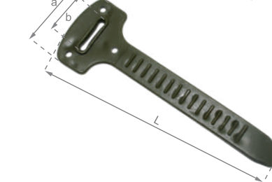
11190 ΛΟΥΡΑΚΙ ΧΑΚΙ ΓΙΑ ΣΤΡΑΤΙΩΤΙΚΟ ΤΖΙΠ KHAKI STRAP FOR ARMY JEEP a=25 / b=20 / L=105
