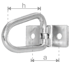
11006 ΠΙ PB ΩΜΕΓΑ ΚΟΝΤΡΑ ΣΠΑΣΤΟ STAPLES PB TIR ROUNDED FOLDED REVERSE a=30 / h=37
