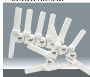
2121 ΠΟΛΛΑΠΛΟ ΚΑΠΟΤΙΝΑΣ AWNING HINGE FOR CANOPY
