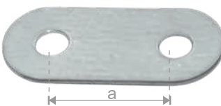
11029 ΡΟΔΕΛΕΣ PB ΓΑΛΒΑΝΙΖΕ ΜΕ ΔΥΟ ΤΡΥΠΕΣ WASHERS PB GALVANIZED WITH TWO HOLES a=20
