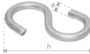
2425 ΣΥΝΔΕΤΙΚΑ S No 40 CLIP S No 40 h=40 / ø3,8
