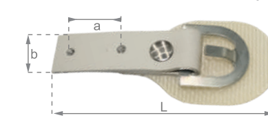
11042 ΤΟΚΑ PB ΚΟΜΠΛΕ ΓΙΑ ΛΟΥΡΑΚΙ COMPLETE PB BUCKLE FOR STRAP a=25 / b=20 / L=105
