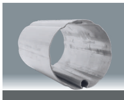
2981 ΣΩΛΗΝΑ ø85 ΚΑΝΑΛΙ ΚΑΙ ΝΕΥΡΟ 6,00M & 6,50M STEEL ROUND TUBE ø85 WITH CANAL 6,00M & 6,50M
