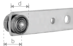
11116 ΡΟΔΑΚΙΑ SA RUNNERS SA b=24 / d=22
