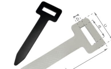
ΛΟΥΡΑΚΙ PB TIR ΜΕ ΟΡΘΟΓΩΝΙΑ ΤΡΥΠΑ STRAP PB TIR WITH RECTANGLE HOLE a=27 / b=8 / c=43 / L=105
