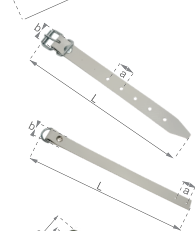
ΛΟΥΡΑΚΙ PB ΜΕ ΤΟΚΑ STRAP PB WITH BUCKLE a=20 / b=20
