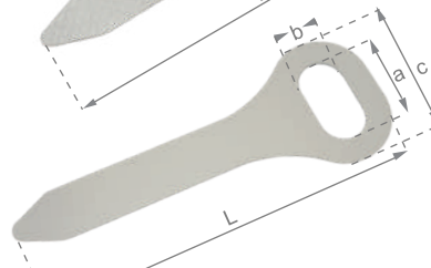
11043 ΛΟΥΡΑΚΙ PB TIR ΜΕ ΣΤΡΟΓΓΥΛΗ ΤΡΥΠΑ STRAP PB TIR WITH ROUNDED HOLE a=42 / b=22 / c=67 / L=180
