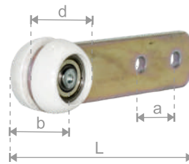
11068 ΡΟΔΑΚΙΑ PB ΓΙΑ ΡΑΓΑ 400 RUNNERS PB FOR RAIL 400 a=29 / b=28 / d=35 / L=125
