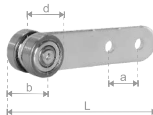
11138 ΡΟΔΑΚΙΑ PB ΓΙΑ ΡΑΓΑ 300 RUNNERS PB FOR RAIL 300 a=29/b=29/d=28/L=124
