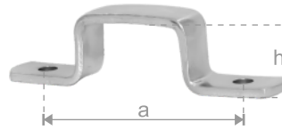
11004 ΠΙ PB TIR ΠΛΑΤΗΣ STAPLES PB TIR PLATE a=57 / h=16
